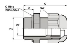
SKINTOP® ST
